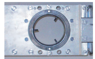
Minimierung des Verschleißes durch konischen Ring mit Bremsrippen
